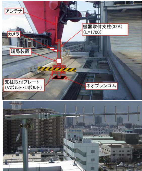
今回設置するアンテナ (上：咲洲庁舎屋上 下：大日通信工業ビル屋上)
