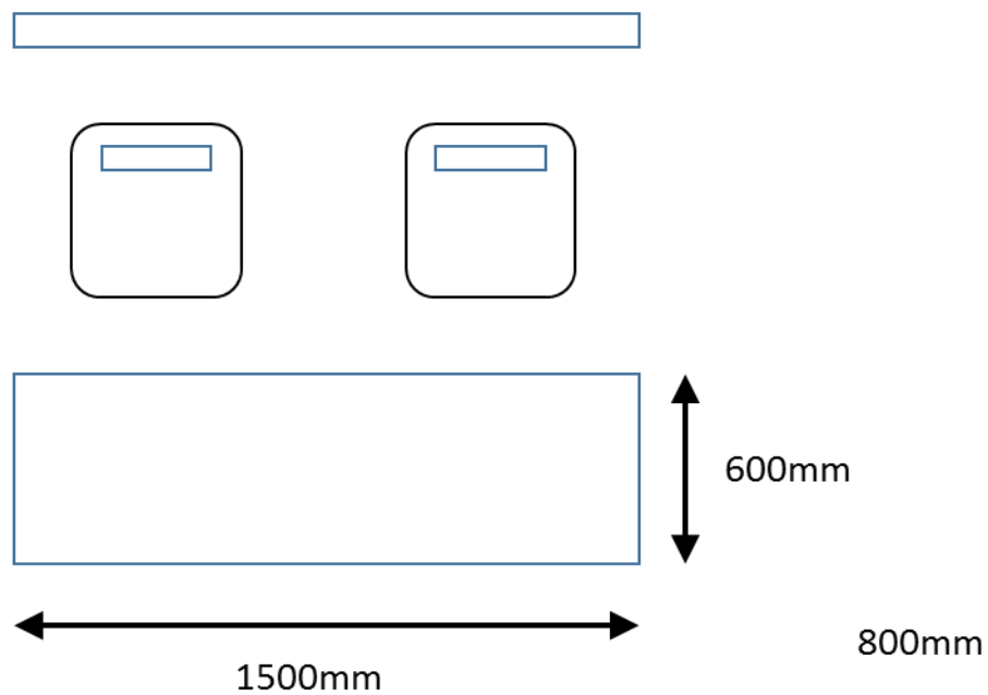
<平面図> (上から見た図)
